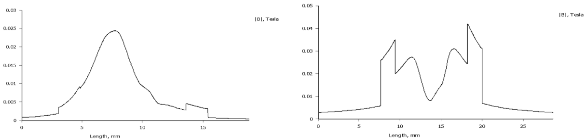
Slika 6.36. Grafički prikaz modula gustoće magnetskog polja NYY kabela za simetrični (desno) i nesimetrični (lijevo) trofazni sustav u trenutku t_3
