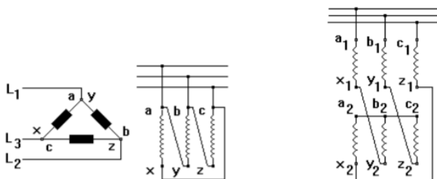
Slika 3.2 Trokut spoj transformator Slika 3.3 Cik-Cak spoj transformatora
