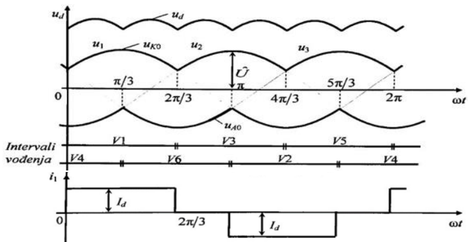
Slika 3.5 Karakteristični valni oblici neupravljivog trofaznog ispravljača [2]
