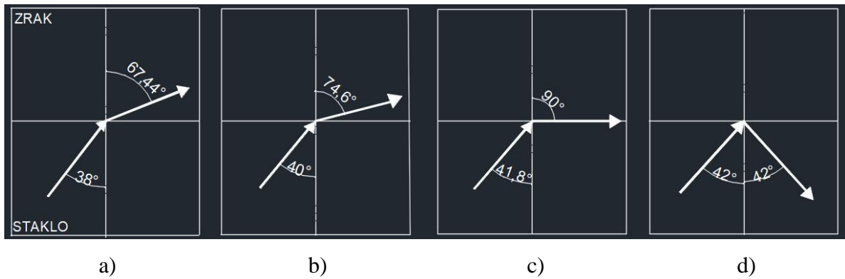
Slika 2.5: Totalna refleksija
