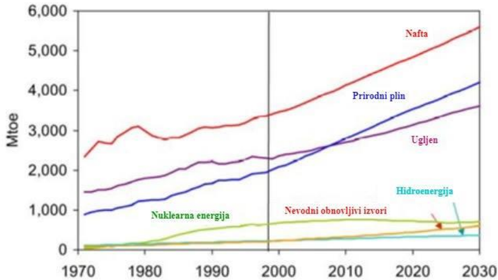
Slika 2.1. Potrošnja primarne energije u svijetu – dosadašnja i predviđanja [3]
