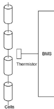
Slika 6.3. Mjerenje temperature termistorom [22]
