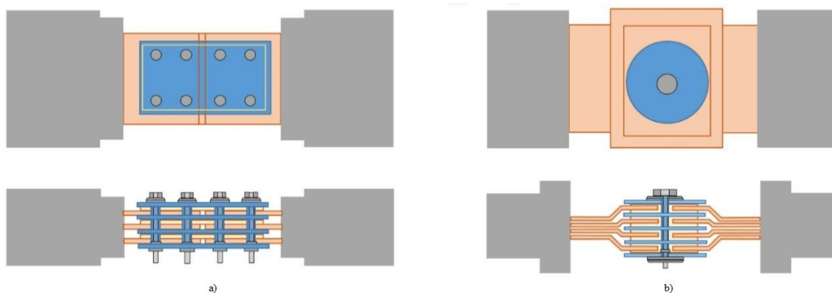
Slika 2.3. Primjeri povezivanja sabirničkih sustava, [5]
