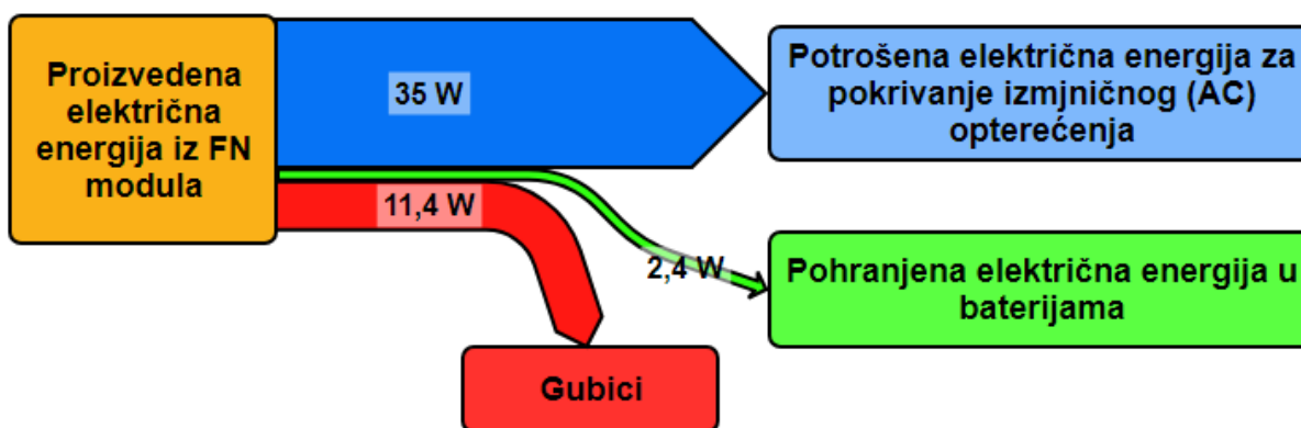
Slika 4.13. Sankey dijagram energetske bilance izmjenično/istosmjernje (AC/DC) mikromreže sa izmjeničnim (AC) opterećenjem [14]
