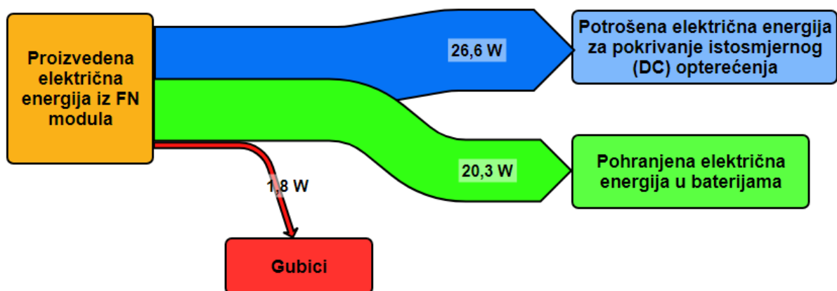
Slika 4.10. Sankey dijagram energetske bilance istosmjerne DC mikromreže [14]
