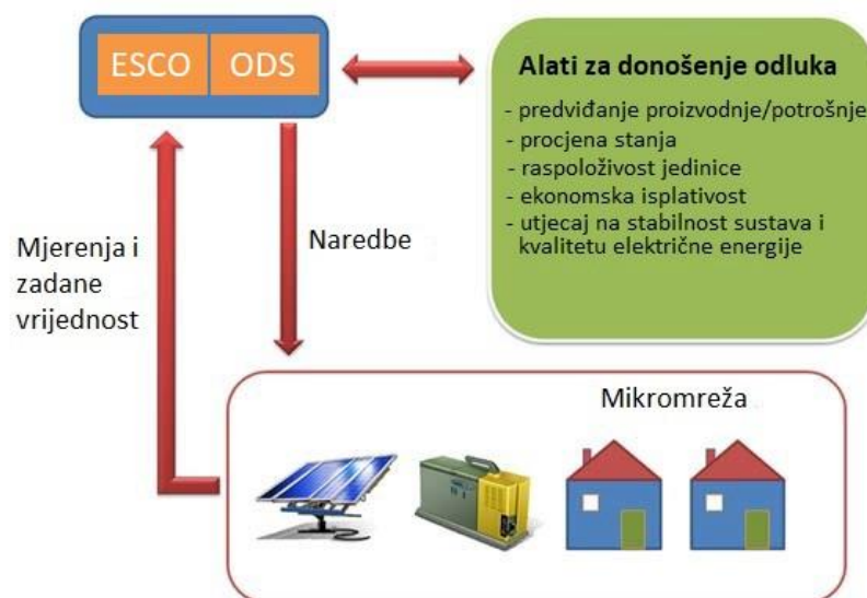
Slika 3.6. Centralizirani način upravljanja [2]
