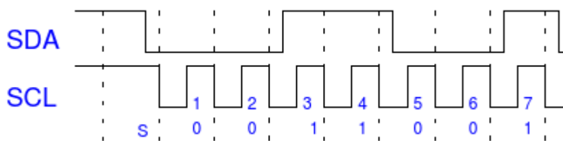
Slika 3.7 I2C komunikacija
