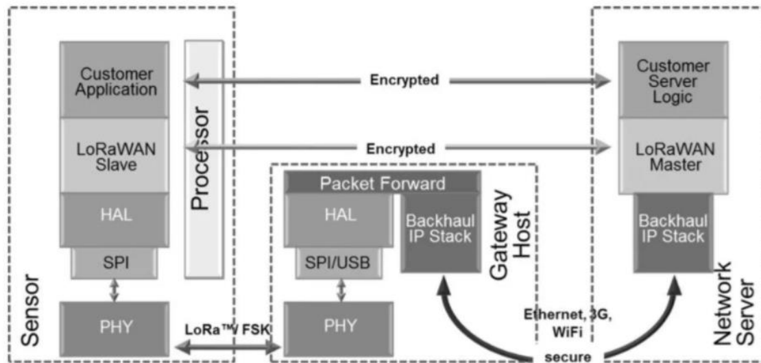
Slika 2.7. LoRaWAN dvoslojna sigurnost [8]
