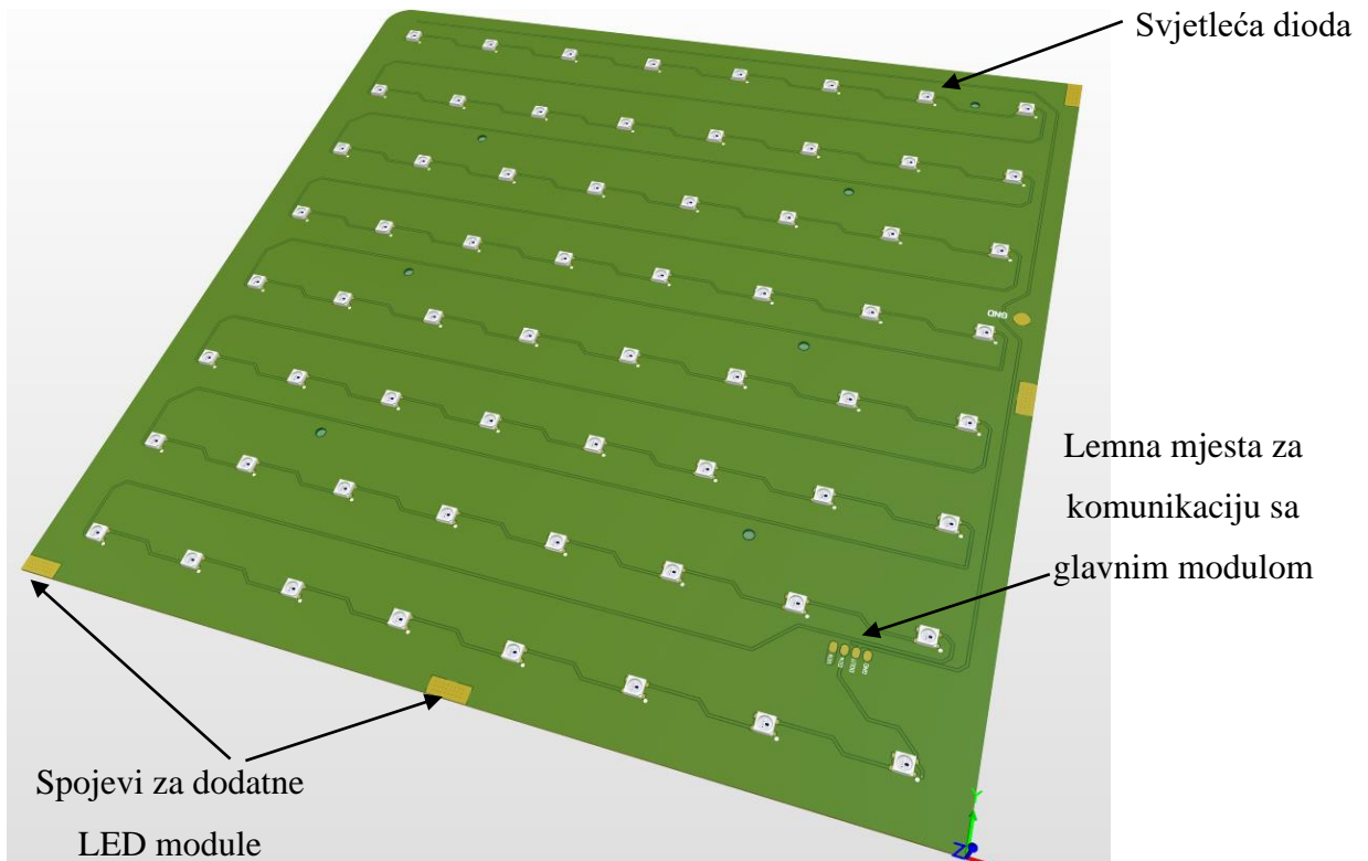
Slika 3.10: LED modul
