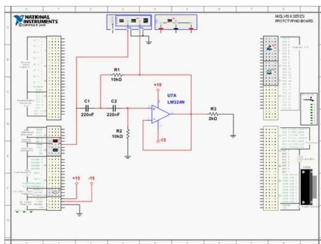
Slika 3.2. Primjer strujnog kruga u Multisim-u s dizajnom NI ELVIS-a II [10]
