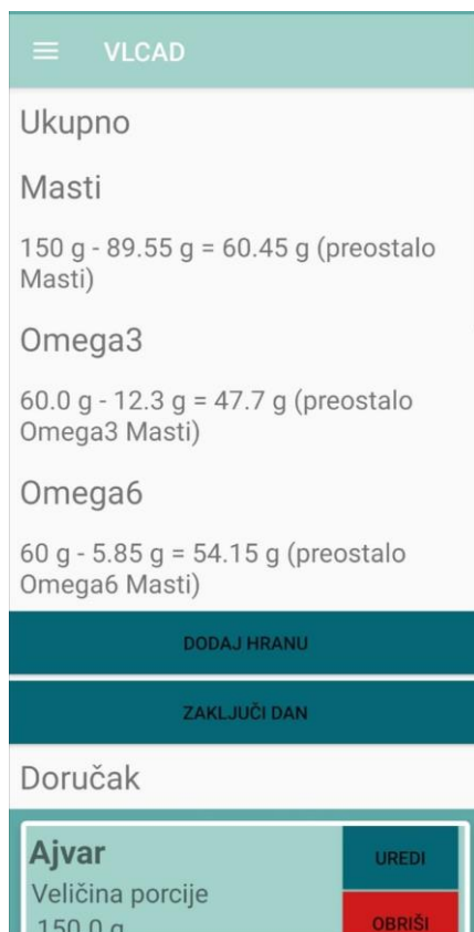
Slika 3.6. Prikaz glavne stranice aplikacije
