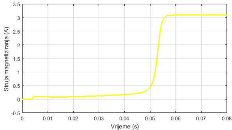
Slika 4.11. Prikaz valnog oblika struje magnetiziranja za U_2 = -36 V
