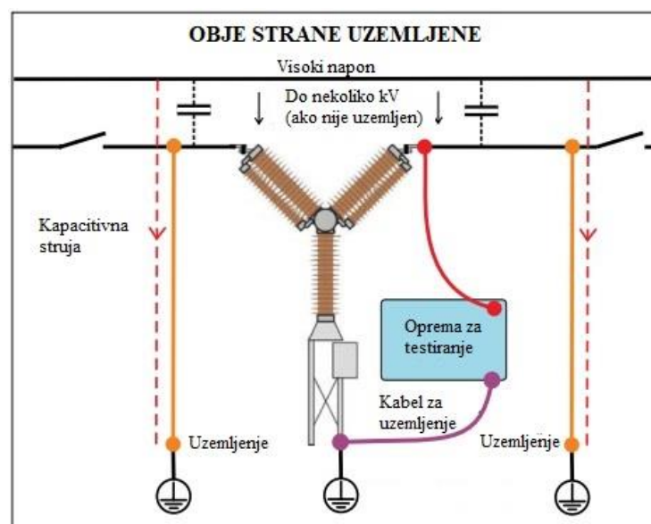
Sl.4.3. Prikaz DualGround ispitivanja
