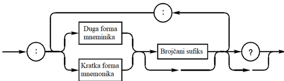
Slika 2.3. Sintaksa naredbi za upravljanje instrumentima
