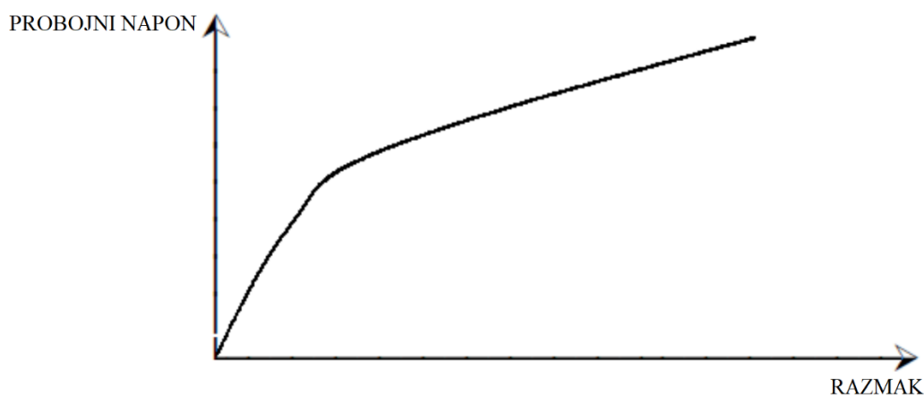
Slika 2.3 Karakteristika probojnog napona mjenog kuglastim iskrištem [2]
