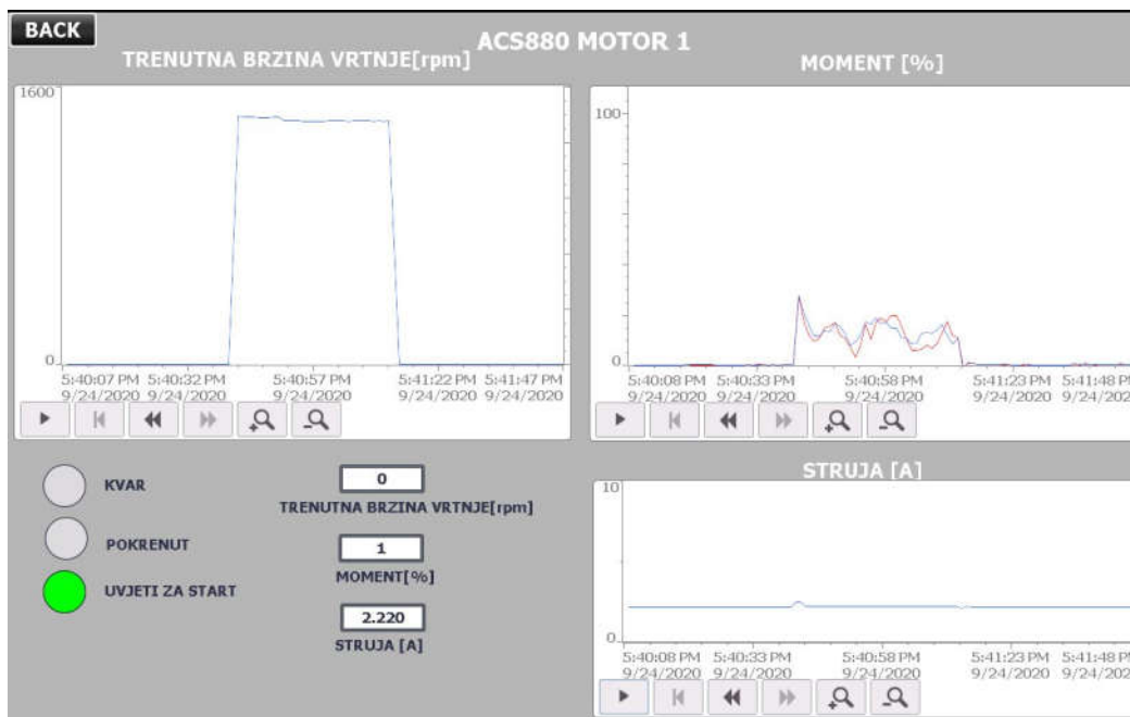
Sl. 6.3. Prikaz procesnih veličina uz Droop
