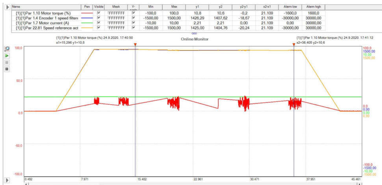
Sl. 6.8. Postupni zalet asinkronog motora na nazivnu brzinu vrtnje
