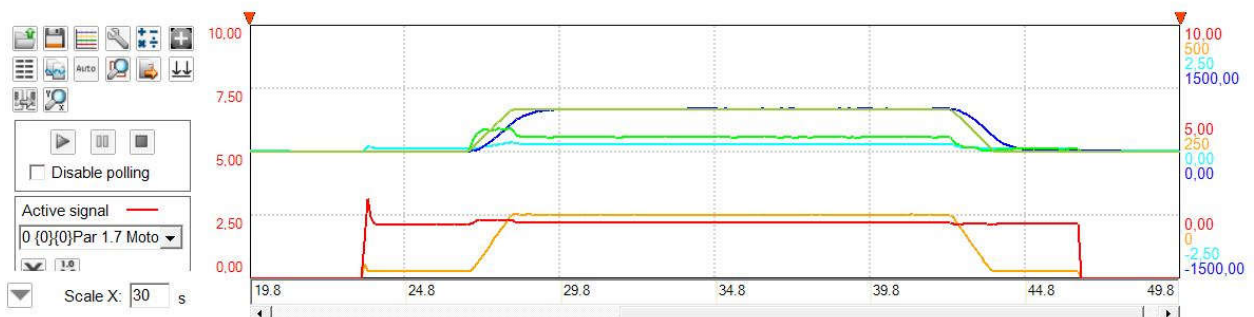
Sl. 4.33. Rampa reference brzine vrtnje sa proporcionalnim pojačanjem K_p=17 i integracijskom komponentom T_i=0.5 s
