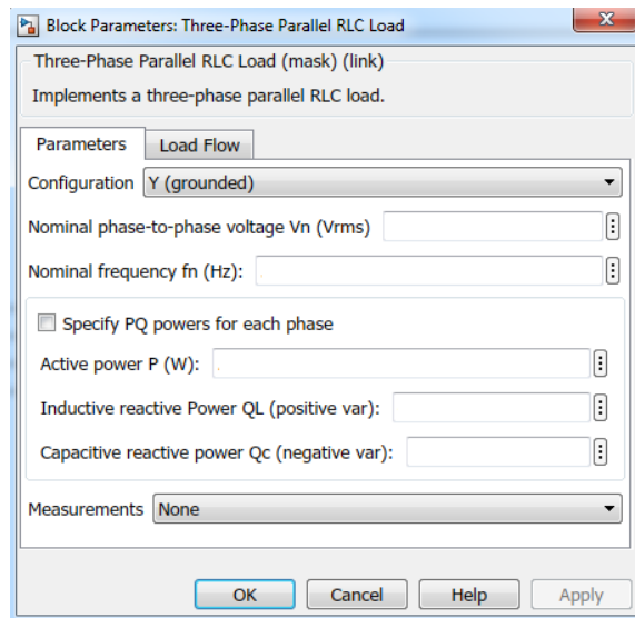
Slika 5.15. Blok za parametriranje potrošača
