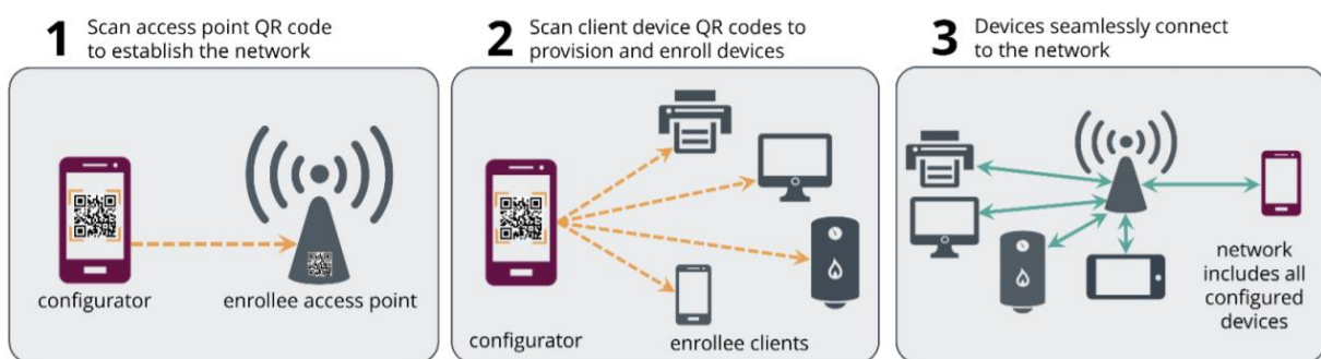
Slika 3.3: Wi-Fi Easy Connect princip rada. [16]
