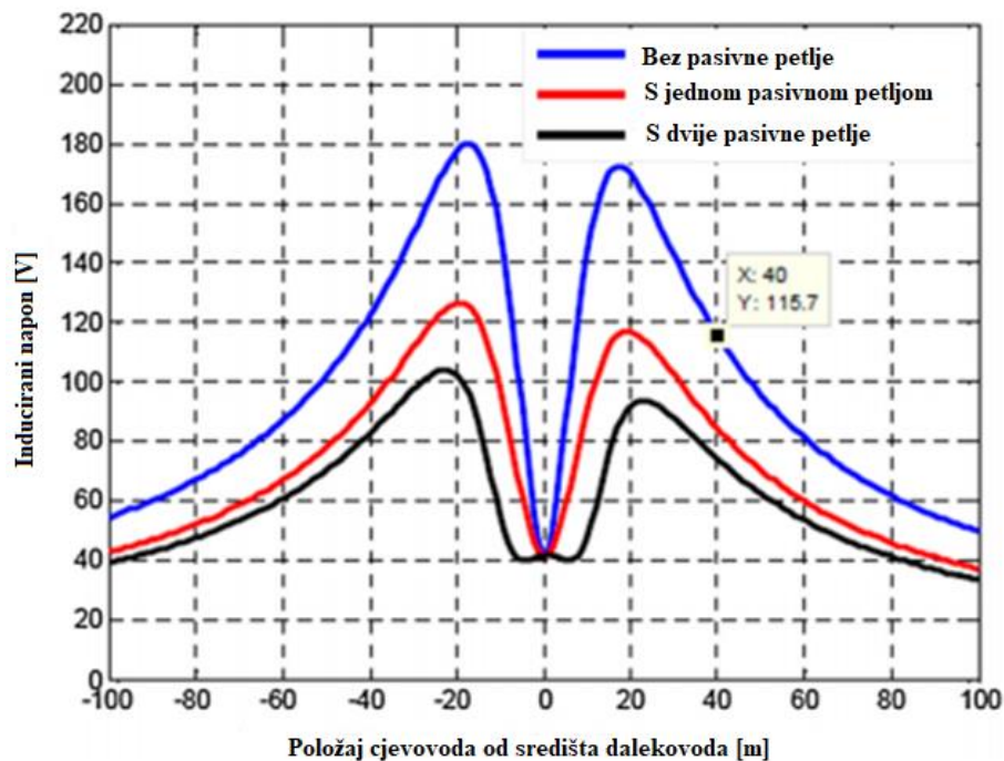
Slika 3.11. Inducirani napon cjevovoda sa i bez pasivnog štita (materijal s relativnom permeabilnosti \mu_r=1 ) [16]
