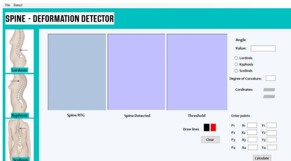
Slika 4.1. Izgled aplikacije
