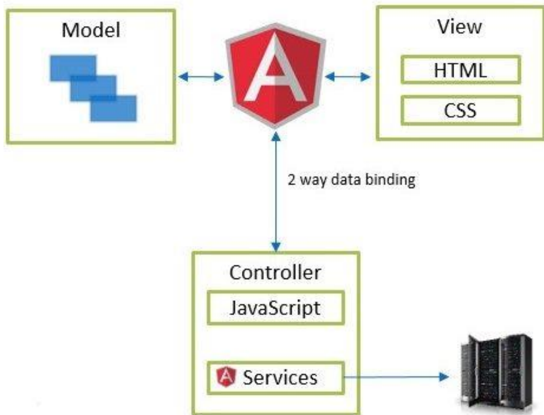
SI. 3.3 Model-pogled-upravljач
