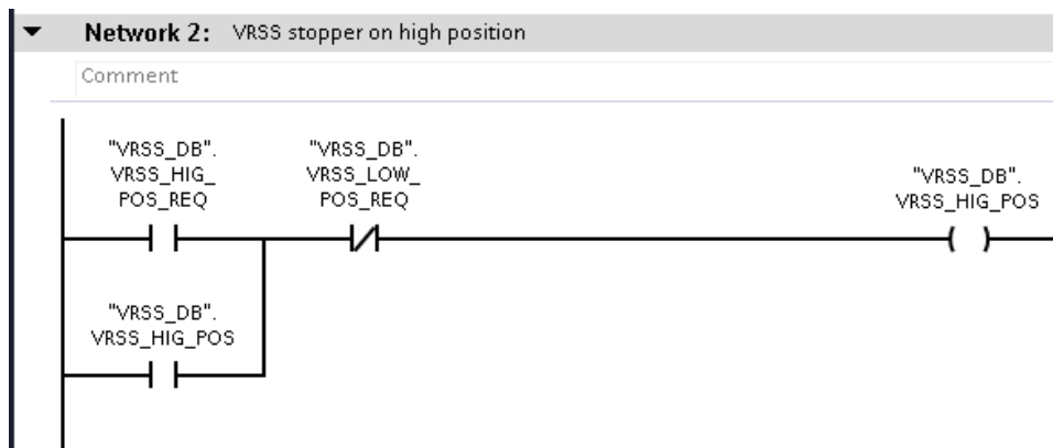
Sl.3.14. VRSS graničnik u gornjoj poziciji
