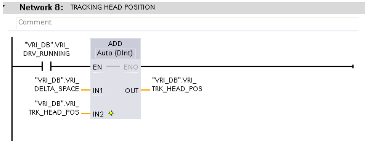
Sl.3.4. Programsko rješenje određivanja prijednog puta na VRI transportnom stolu
