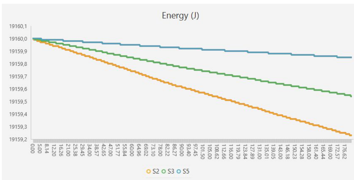
SI.2.10. Razina energije nakon simulacije u čvorovima S2 (100%), S3 (60%) i S5 (20%) pri jednakoj udaljenosti
