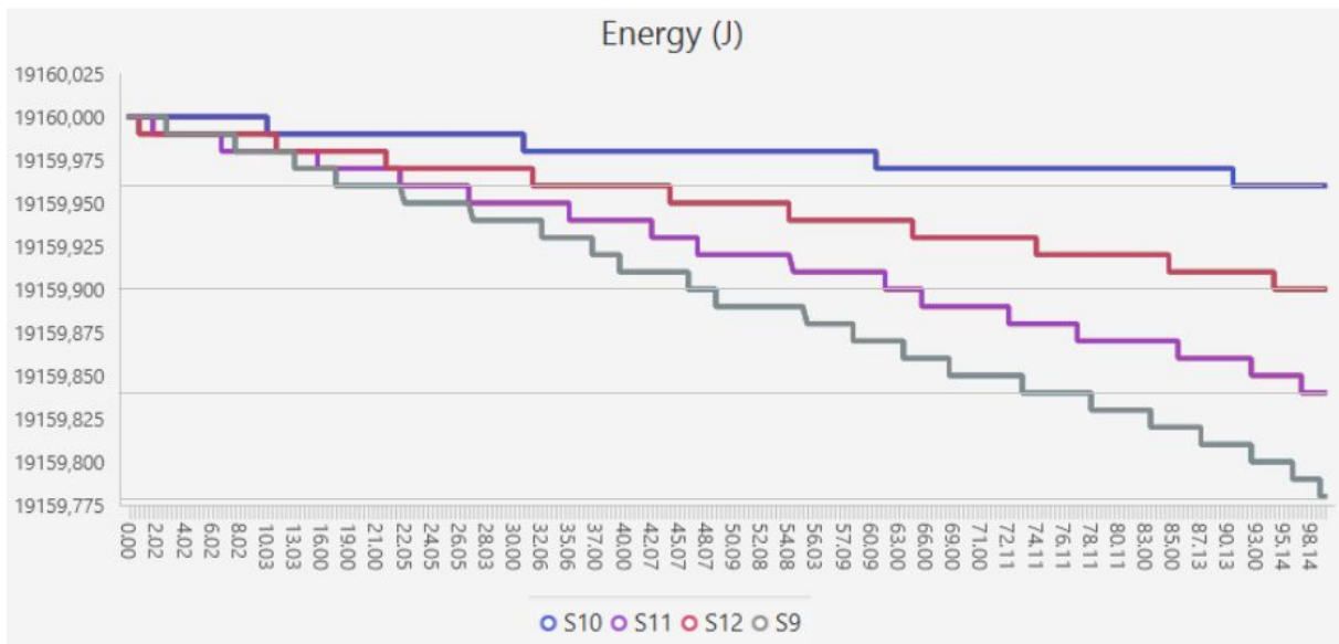
Sl.3.16. Razina energije nakon simulacije za primjer 2.a)
