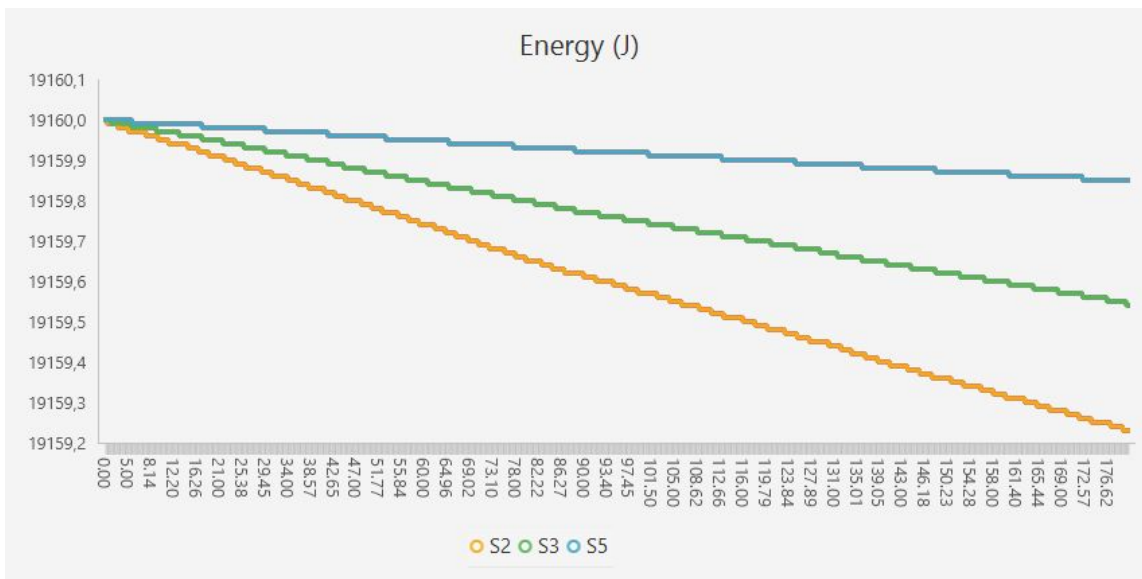
Sl.2.10. Razina energije nakon simulacije u čvorovima S2 (100%), S3 (60%) i S5 (20%) pri jednakoj udaljenosti
