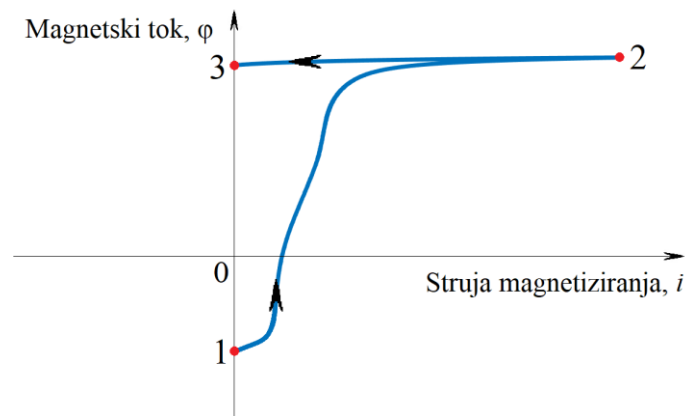
Slika 1.6. Postupak predmagnetiziranja prikazan u \varphi - i ravnini.
