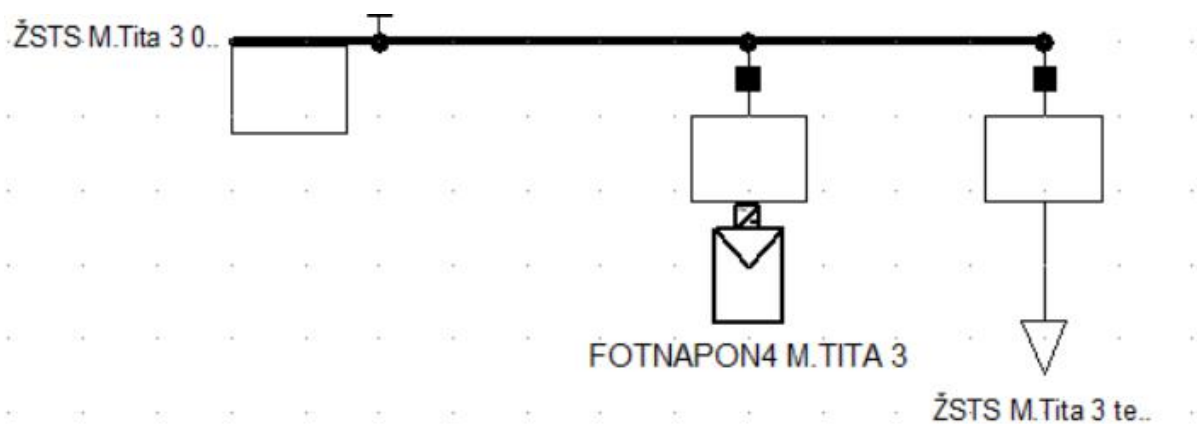
Slika P.3. Prikaz fotonaponske elektrane na sabirnici Vodocrpiliste
