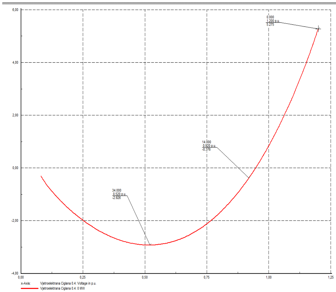
Slika 4.13. Q-V krivulja nakon povećanja opterećenja
