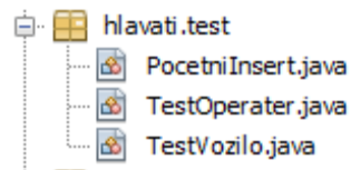
Slika 4.5 Paket test
