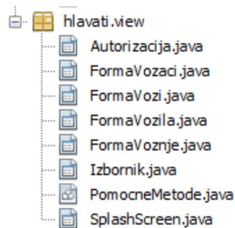
Slika 3.4. View aplikacije
