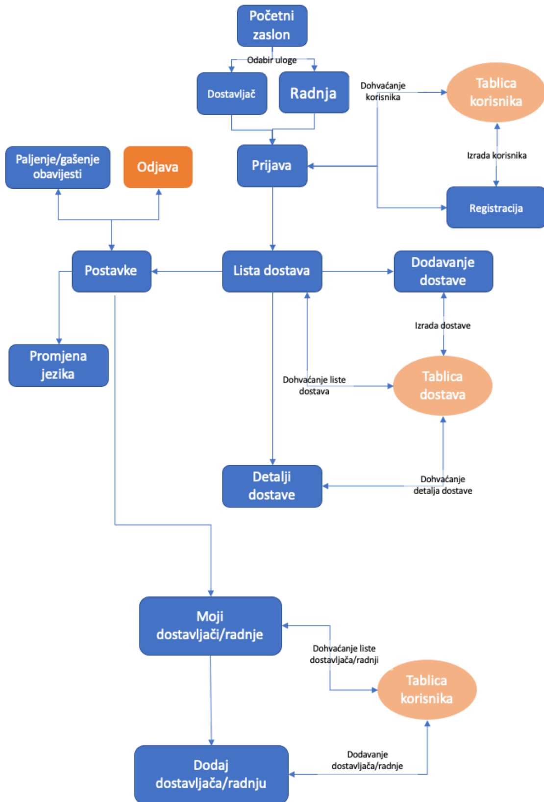
Slika 3.1 Model aplikacije.
