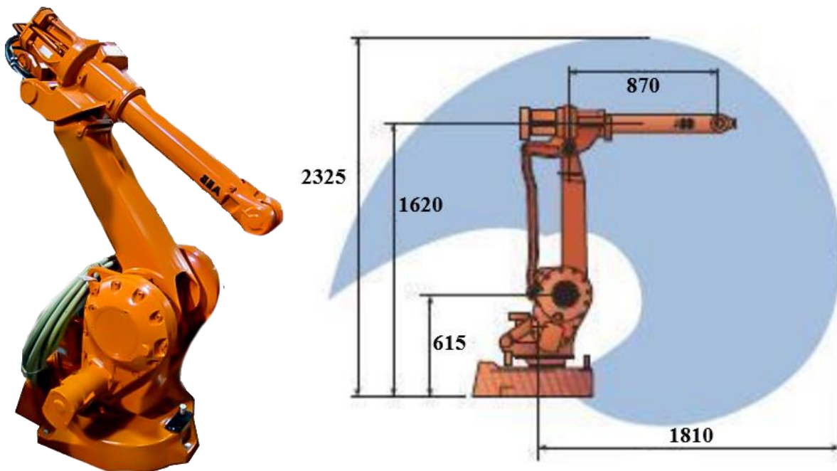
Slika 4.1. Industrijski robotski manipulator IRB 2400L (lijevo); Dimenzije manipulatora IRB 2400 L (desno)
