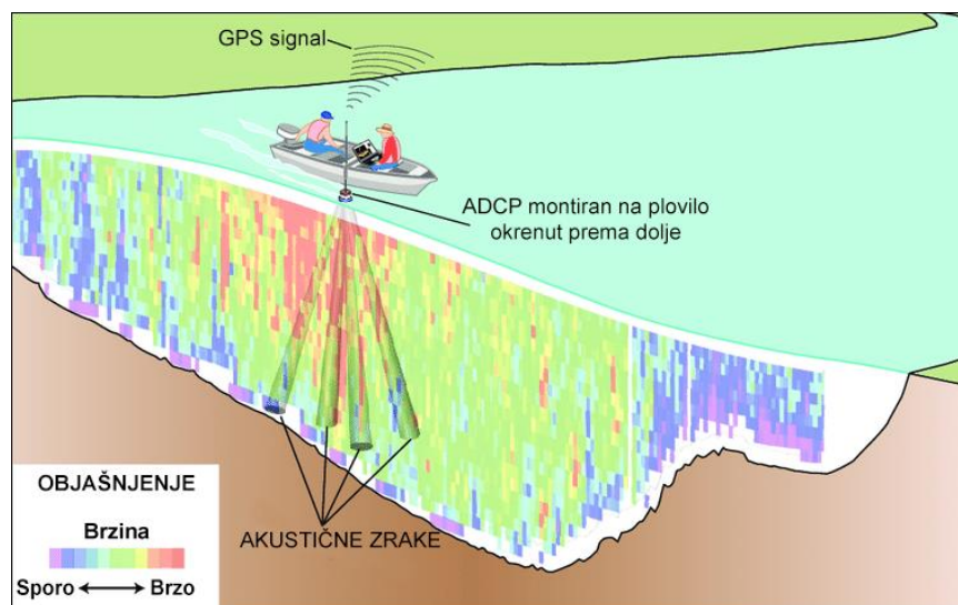
Slika 5.2.3. Objašnjenje metode mjerenja brzine vode ADCP-om [32]
