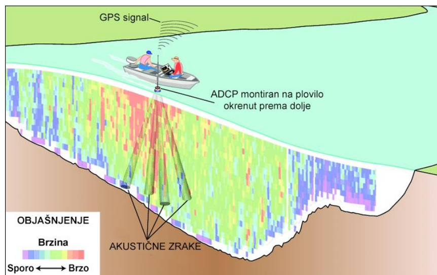
Slika 5.2.3. Objasnjenje metode mjerenja brzine vode ADCP-om [32]
