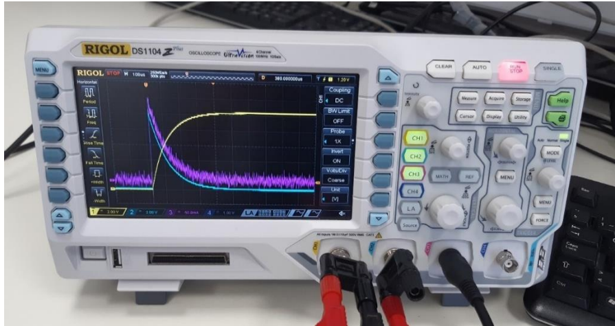
Slika 4.3. Osciloskop
