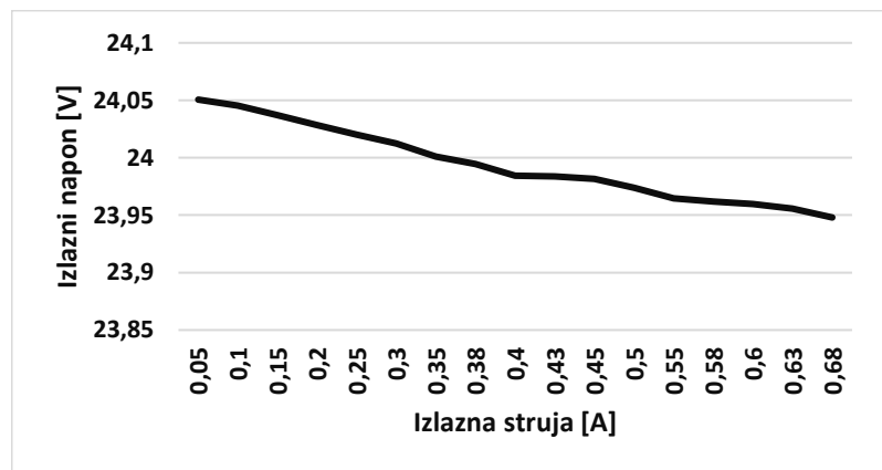
Sl. 5.9. Graf ovisnosti izlaznog napona o povećanju izlazne struje za vrijednost izlaznog napona 24V.
