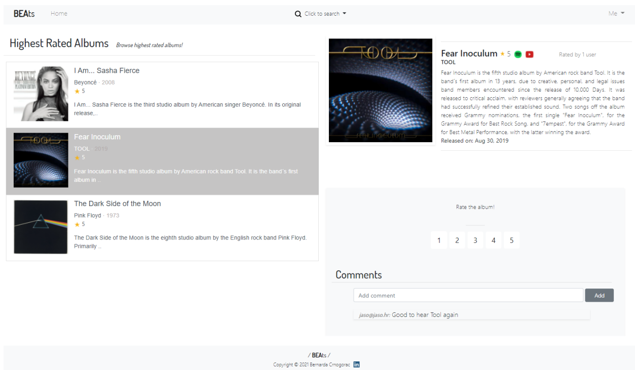
Slika 4.12. Album-detail-highest komponenta
