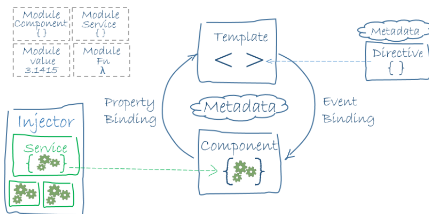
Slika 2.1. Arhitektura Angular aplikacije
