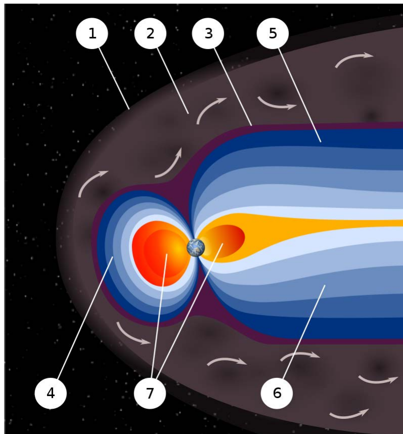
Slika 12 Dijelovi magnetosfere.
