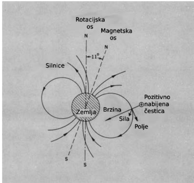
Slika 7 Magnetsko polje Zemlje, nagnuto 11^\circ u odnosu na os rotacije. Točna lokacija magnetskih polova varira vremenom. Dolazeća pozitivno nabijena čestica bit će prisiljena promijeniti putanju kako je prikazano na slici. [1]
