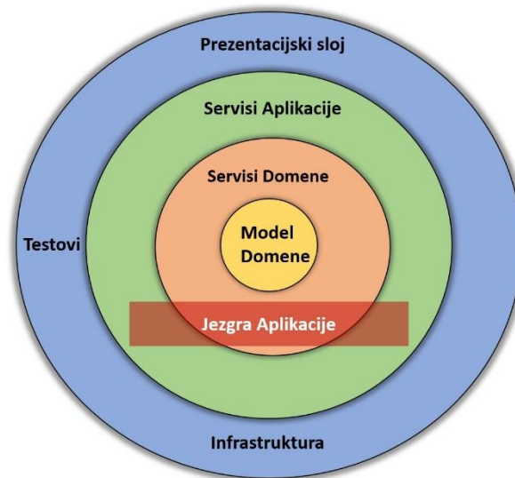
Slika 4.6. Onion arhitektura
