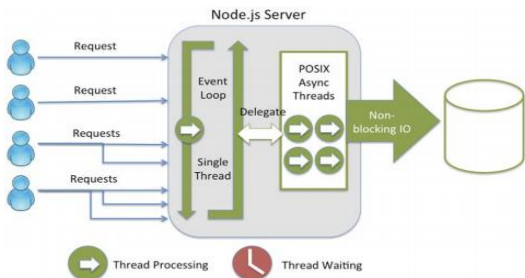
Slika 3.5. Node.js arhitektura.[5]
