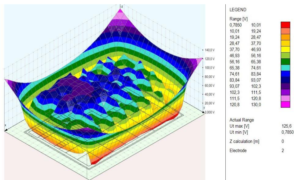
6.36. 3D prikaz napona dodira s obzirom na ogradu, oграда galvanски odvojena
