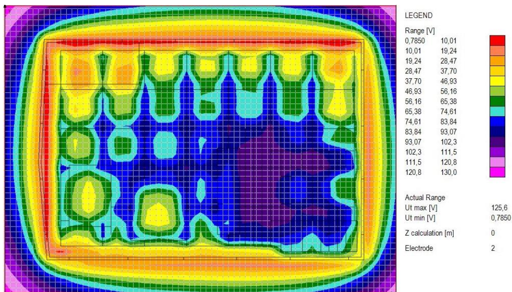
Slika 6.35. 2D prikaz napona dodira s obzirom na ogradu, oграда galvanски odvojena
