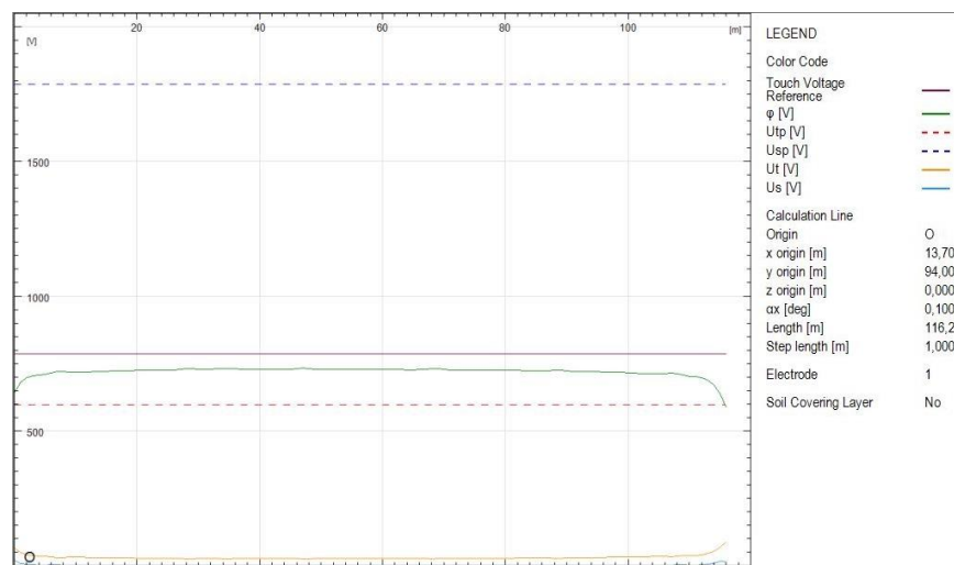
Slika 6.50. Graf napona dodira i koraka uz istočnu ogradu na udaljenosti 1m, oграда galvaniski spojena
