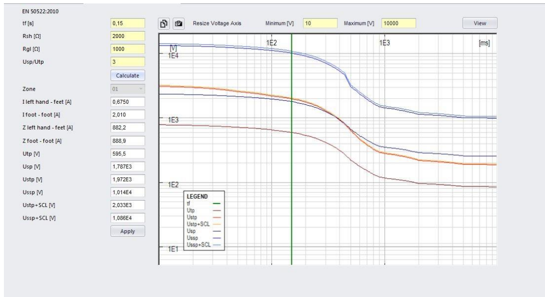
Slika 6.29. Dopuštene vrijednosti napona dodira i koraka prema europskom standardu
