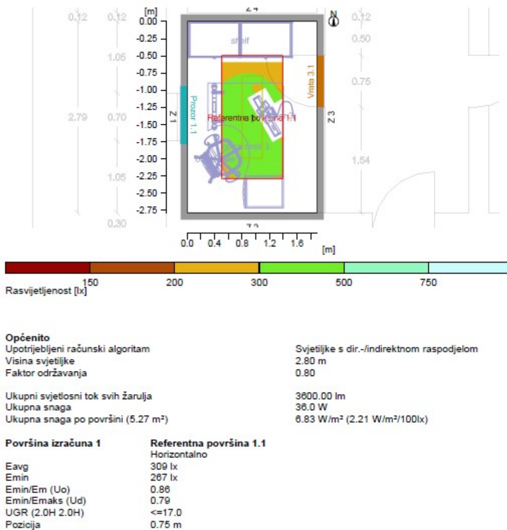
SI.6.8. Prikaz rasvjetljenosti uredskog prostora
