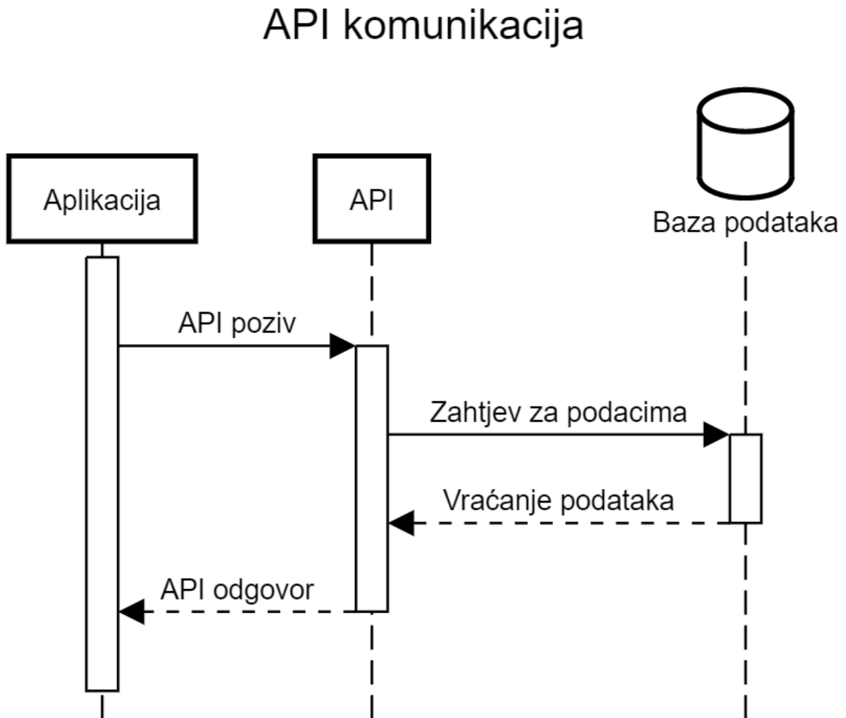
Slika 3.1.: Sekvencijalni dijagram API komunikacije
