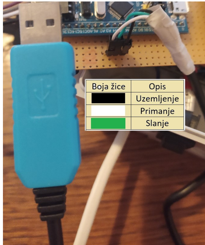
Sl. 3.5. Povezivanje PL2303TA pretvornika.
