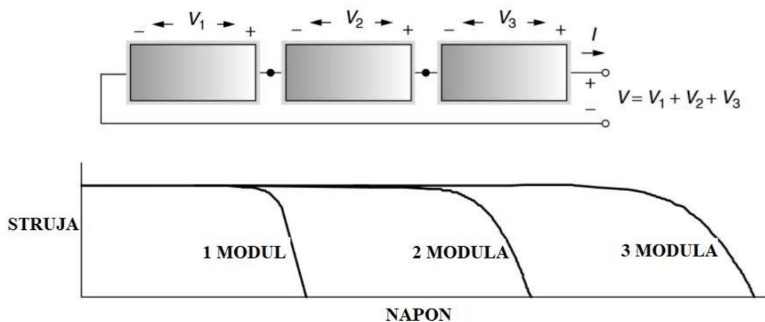
Sl. 3.4. Strujno-naponska karakteristika modula u serijskom spoju. [1]
