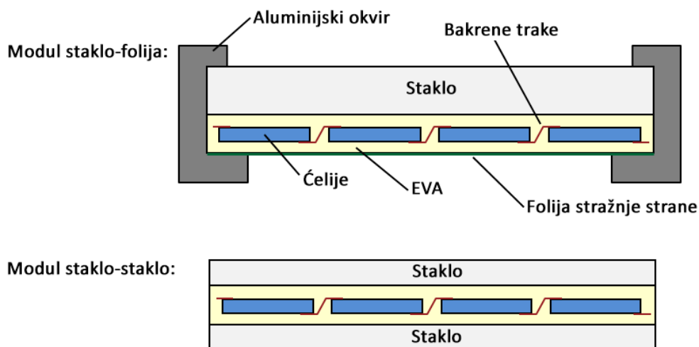
Sl. 2.2. Presjek monosilicijskog fotonaponskog modula [3]
