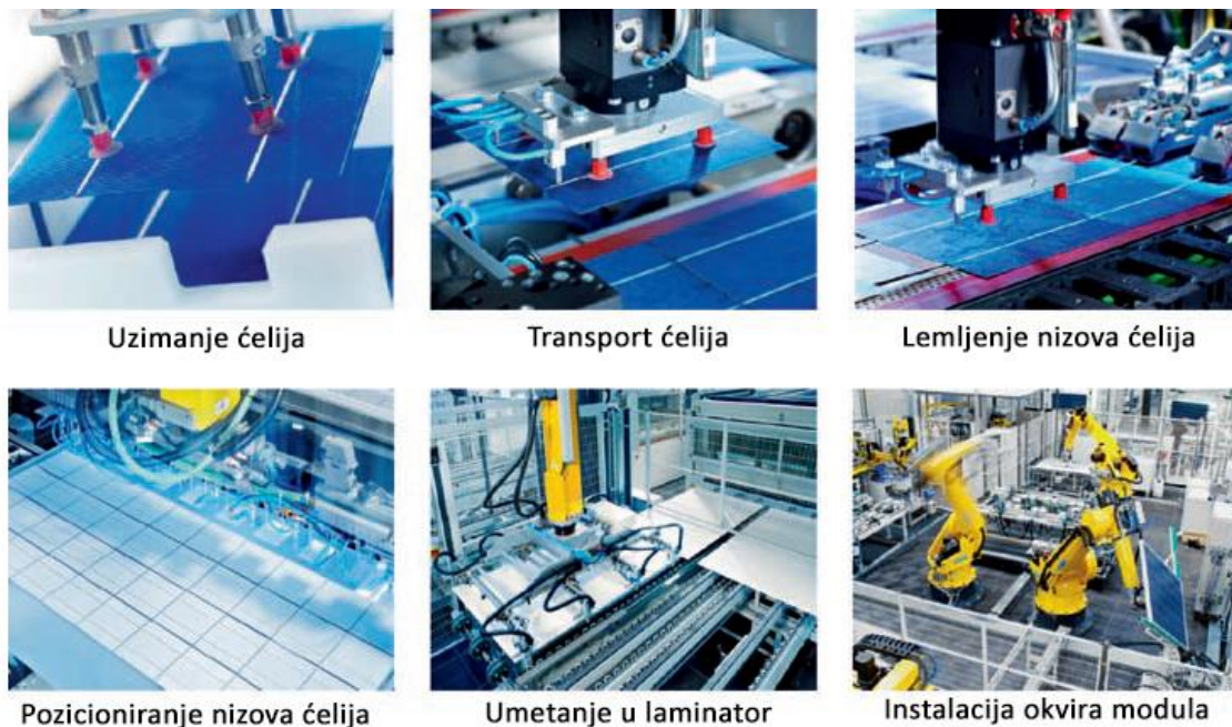
Sl. 2.3. Koraci proizvodnog procesa fotonaponskog modula (izvor: Solar-Fabrik AG) [3]
