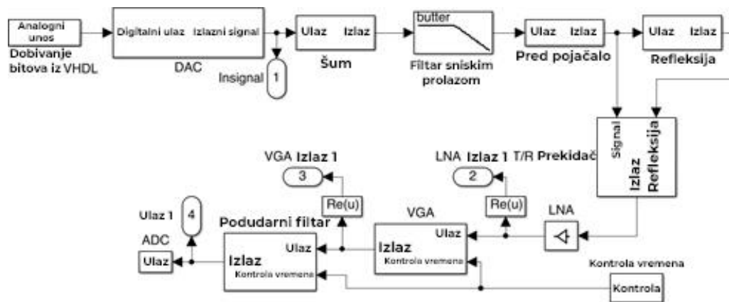
Sl. 5.1. Blok shema analognog modela za svaku komponentu pri uvozu podataka iz VHDL-a [12]
