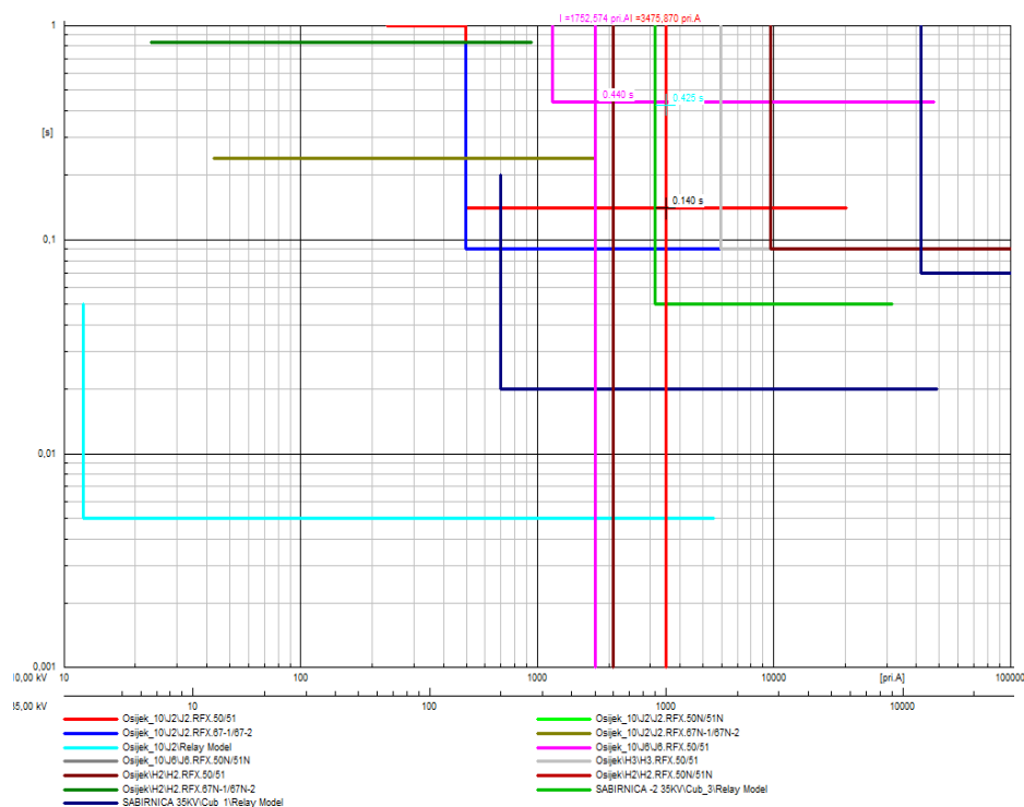
Slika 6.22. Koordinacija mreže za trolezni kratki spoj
