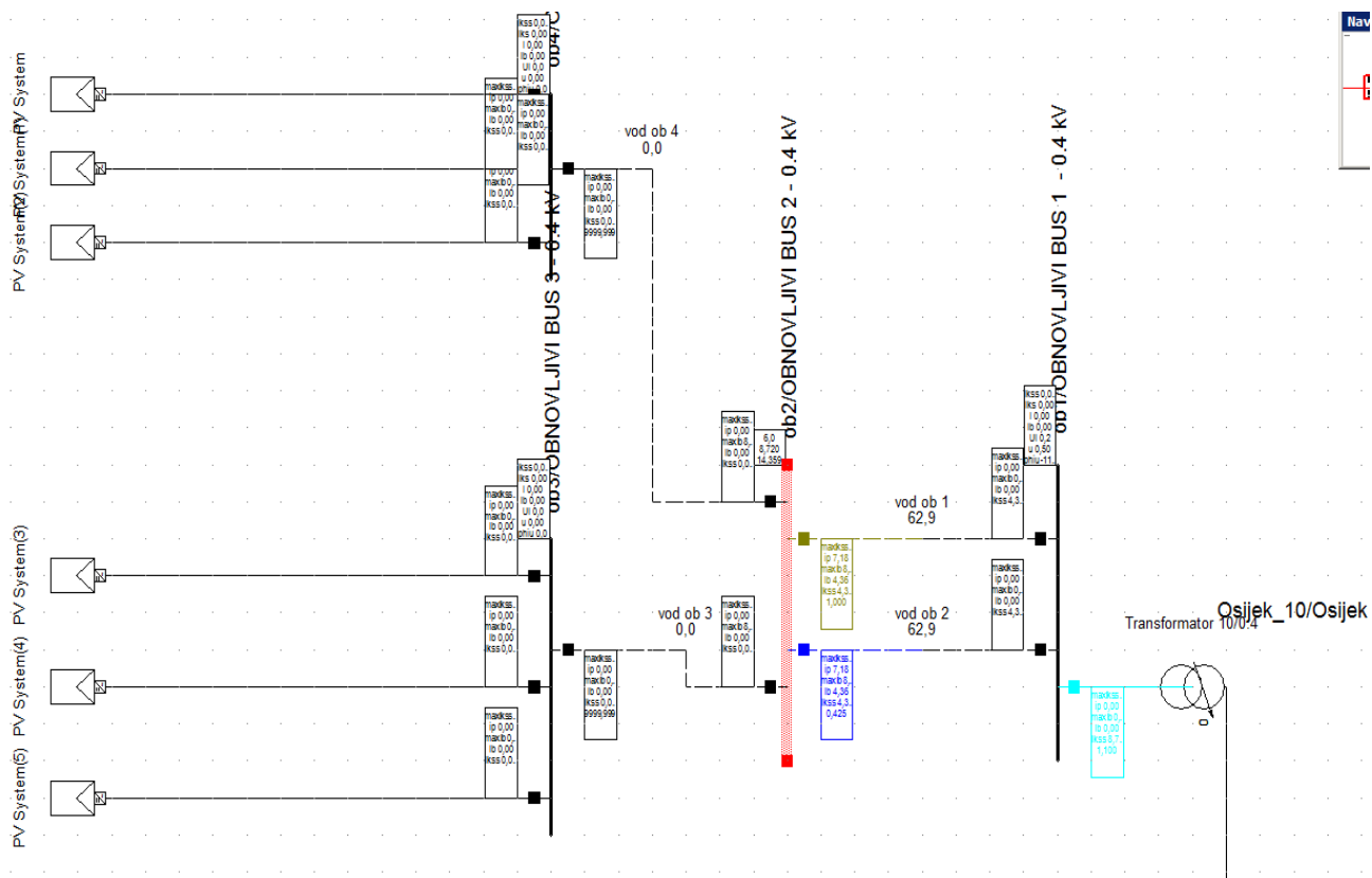
Slika 6.12. Lokacija releja PR512/Px (50-51 50N-51N) (plavi desno)
