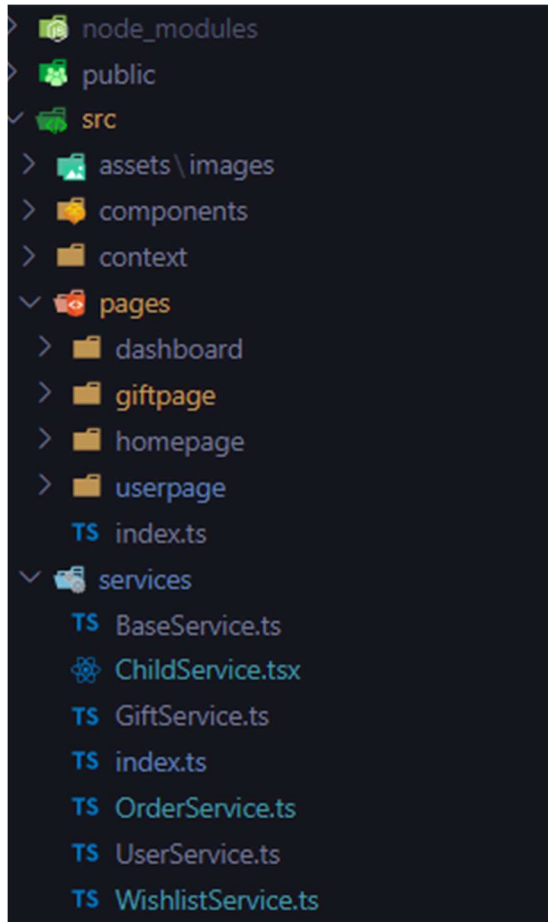
Slika 5.3. Struktura direktorija.
