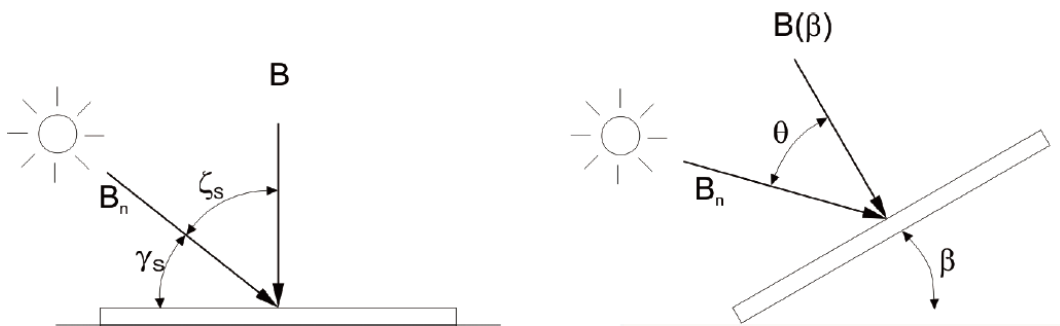
Slika 2.3. Izravno zračenje na vodoravnu i nagnutu plohu [12]
