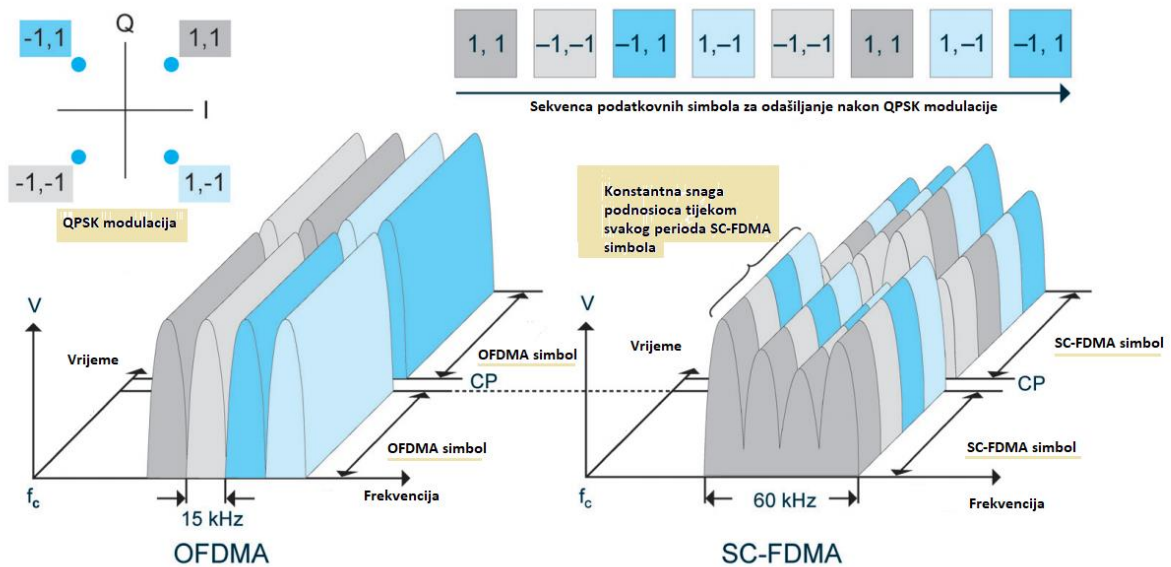
Slika 3.12. Usporedba između prijenosa QPSK simbola primjenom OFDMA i SC-FDMA [19]
