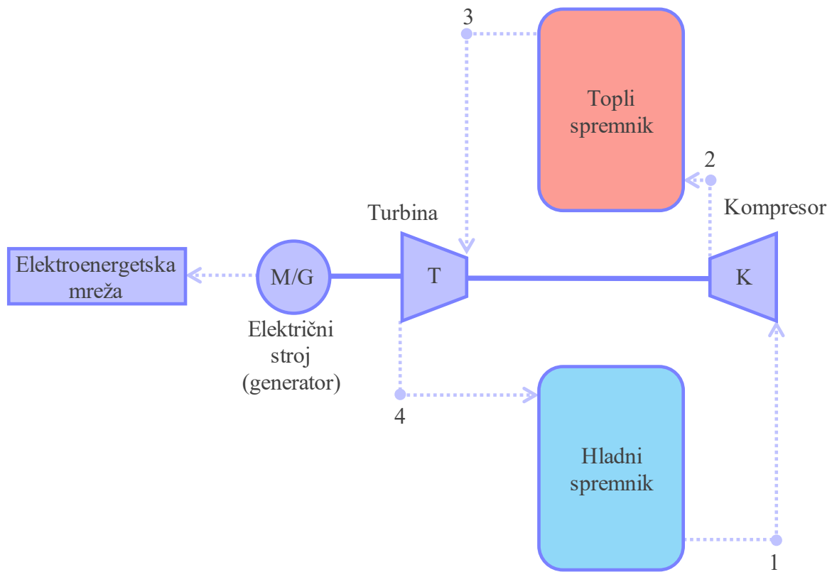
Sl. 3.7. Korištenje pohranjene električne energije reverzibilne toplinske pumpe [16]
